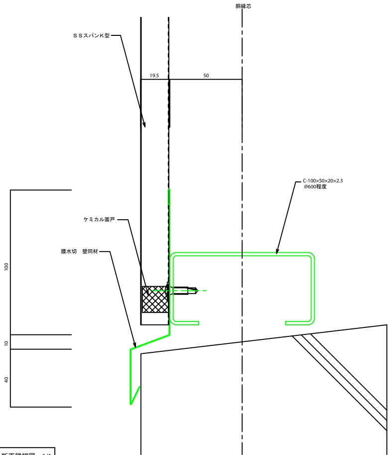
腰水切 断面詳細図 1/1
